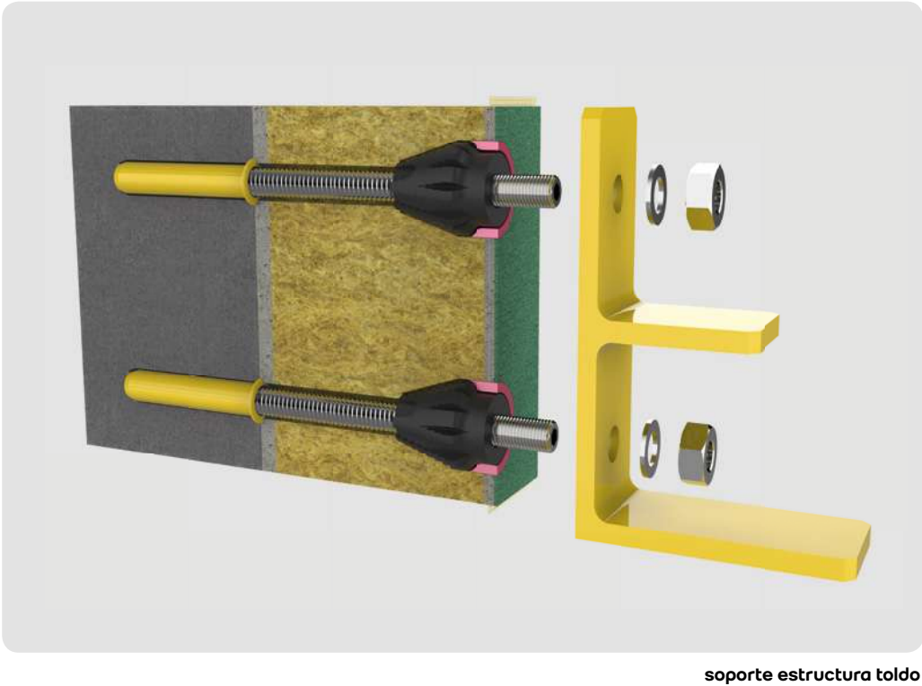
soporte estructura toldo
