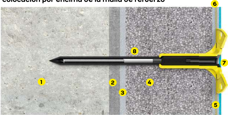
colocación por encima de la malla de refuerzo
